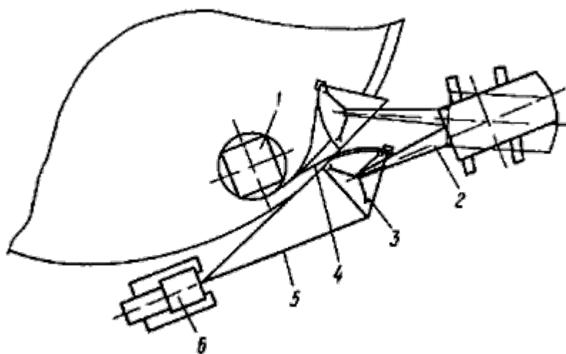
1 - рулон стенки; 2 - кран; 3 - гибочный сектор; 4 - формобразуемый участок полотна; 5 - тяговый канат; 6 - трактор
