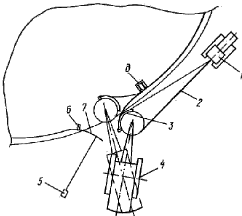
1 - трактор; 2 - тяговый канат; 3 - приспособление для формообразования; 4 - кран; 5 - наземный якорь; 6 - упор; 7 - формобразованный участок полотна; 8 - стойка-упор
