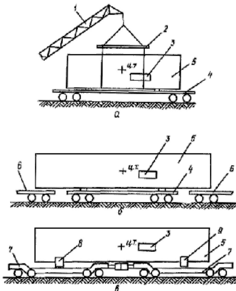
1 - самоходный кран; 2 - разгрузочная траверса; 3 - место маркировки рулона; 4 - четырехосная железнодорожная платформа; 5 - рулон; 6 - платформа прикрытия; 7 - сцепной транспортер; 8 - неподвижный ложемент; 9 - подвижный ложемент
