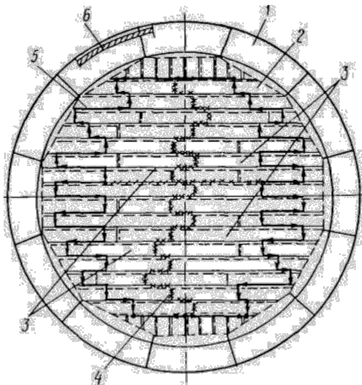
1 - окрайка; 2 - периферийные листы; 3 - зона; 4 - шов между зонами; 5 - шов между периферийными листами и зонами; 6 - стенка
