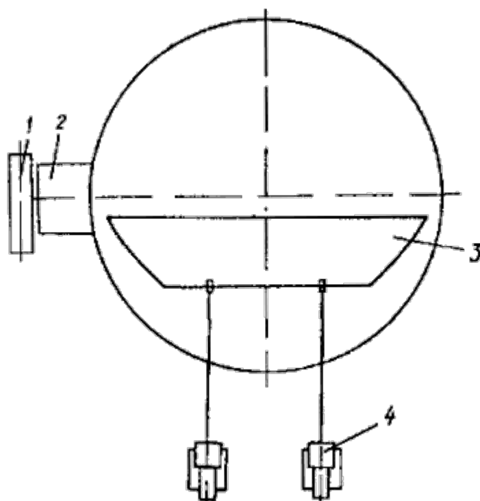
1 - исходное положение рулона днища; 2 - пандус; 3 - развернутое полотнище; 4 - трактор
