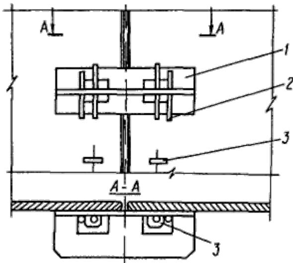
Сборка вертикального стыка между листами стенки
