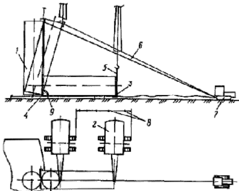
Подъем рулона стенки краном, перемещающимся в процессе подъема
