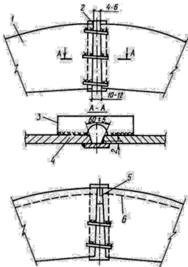
Схема сварки стыков окрайек
