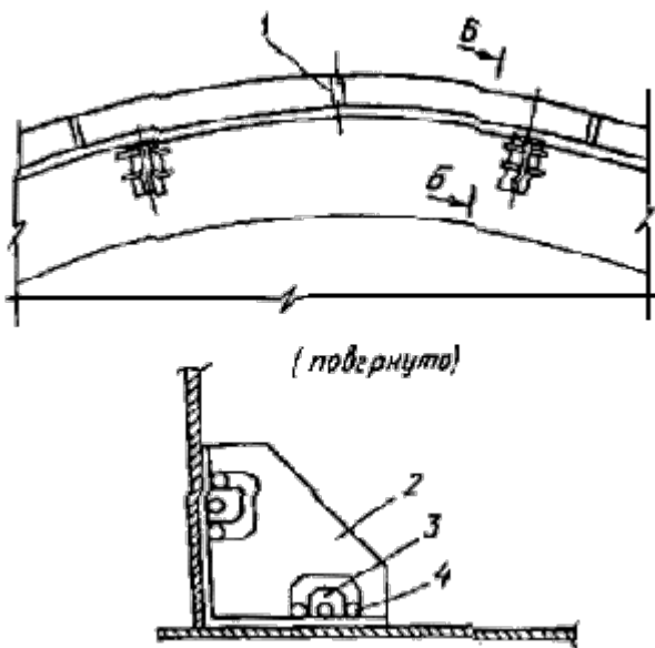
Сборка листов первого пояса стенки с днищем
