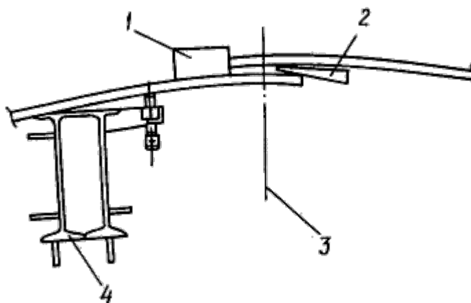
Замыкание вертикального монтажного стыка
