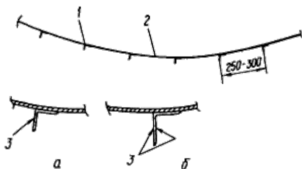
1 - ограничительный уголок; 2 - стенка резервуара; 3 - приварка
