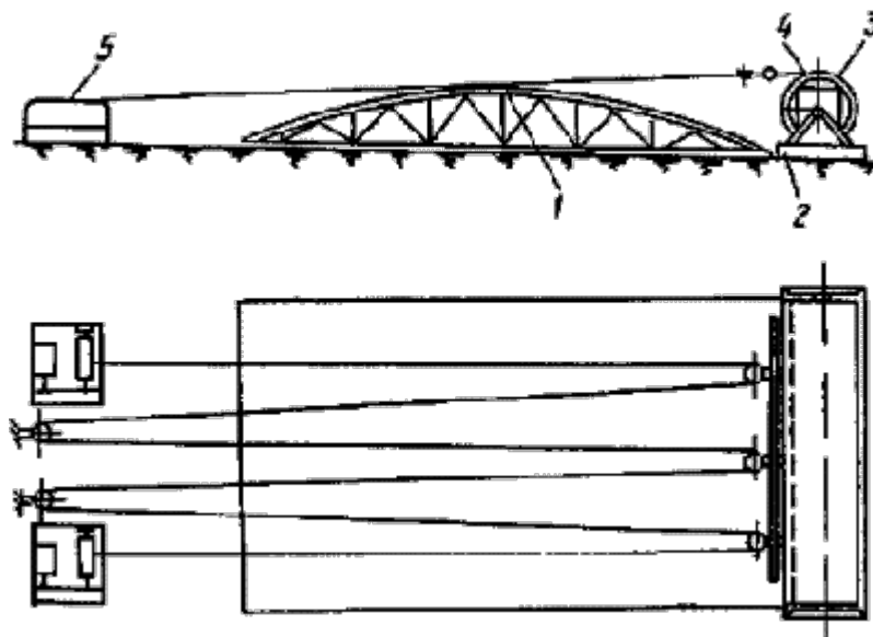
1 - стенд; 2 - опора; 3 - рулон; 4 - полотнище стенки; 5 - электрические лебедки
