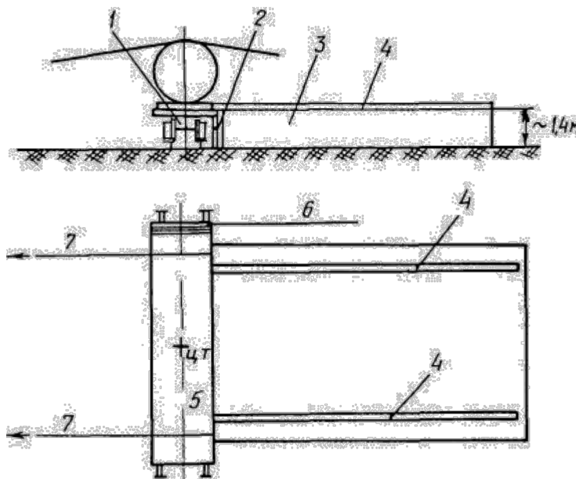
Разгрузка рулона на рампу для приема и хранения рулонов
