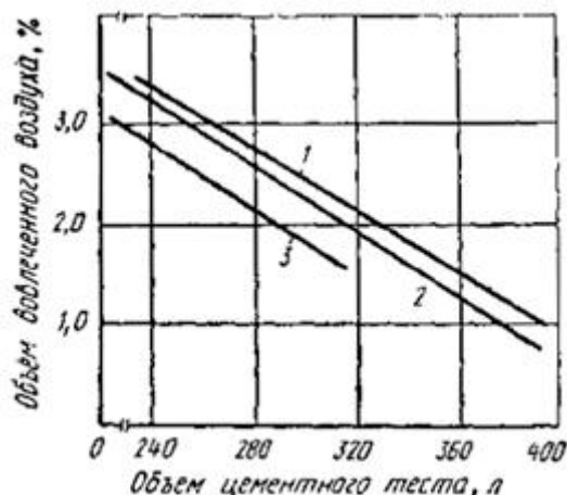
Рис. 2. Количество вовлеченного воздуха в бетонной смеси с добавкой силиконата натрия в зависимости от объема цементного теста с наибольшей крупности щебня:
