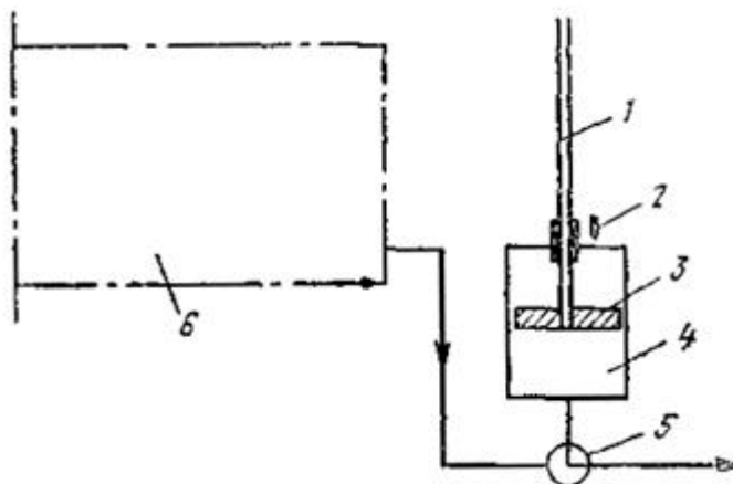
Рис. 2. Схема дозатора ПКБ ЦНИИС:
